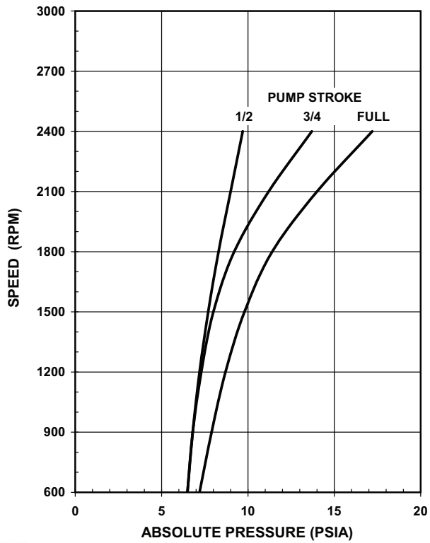
■ PVG-150
